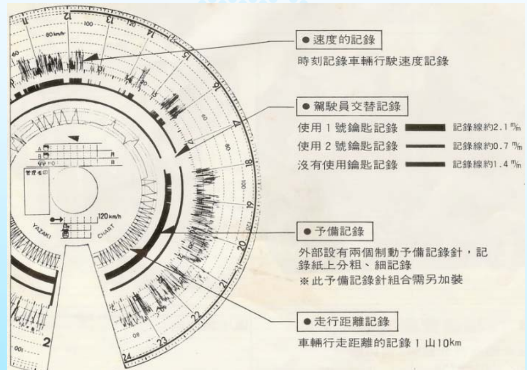
行車紀錄器錄紙-俗稱大餅
